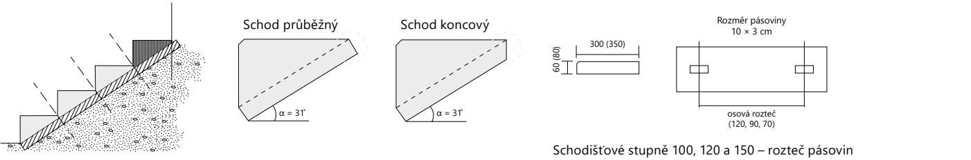
Schodišťové stupně 100, 120 a 150 – rozteč pásovin
