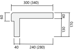
Obklad L typ vnější
